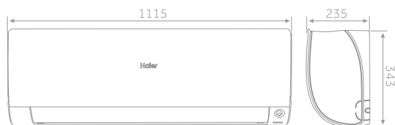
INSTALAČNÍ ROZMĚRY
